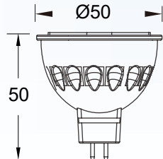
Base Type : GU5.3
